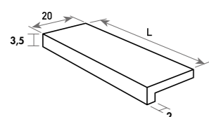
BORDE 3 EDGE 3 20xL 20x61 / 20x76 / 20x120
