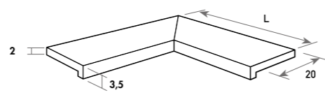
BORDE ÁNGULO INTERIOR 20xL INSIDE CORNER EDGE 20xL 20x61 / 20x76 / 20x120
